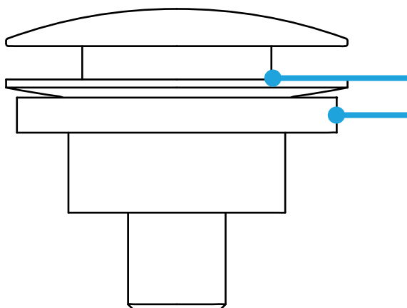
Ablaufgarnitur mit Druckstopfen und Pop-up-Mechanik
